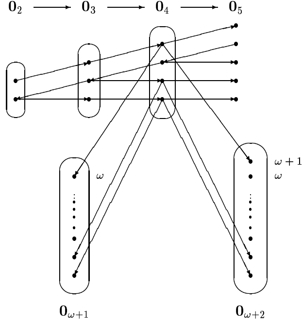
Fig. 1: Counterexample
