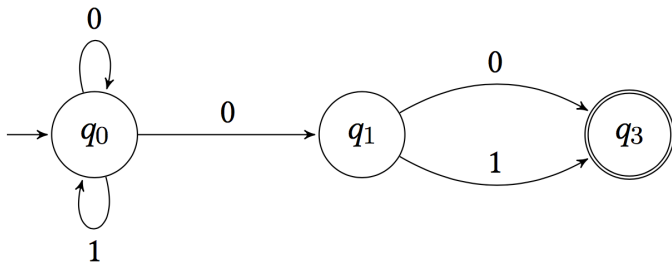
Riconoscitore per (0|1)^*0(0|1)
